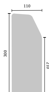
Upotettava J-reunakivi
