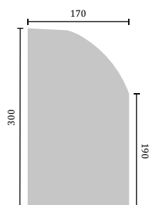
Upotettava H-reunakivi
