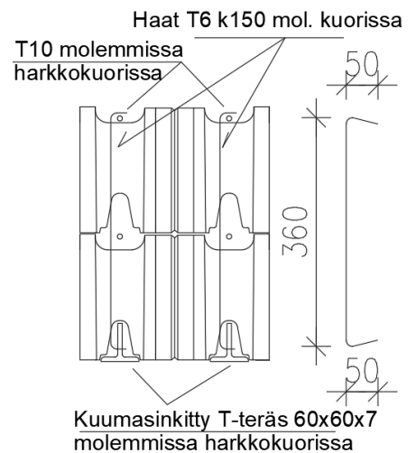
Kuva 6. Liittopalkki EMH-300 harkoilla.
