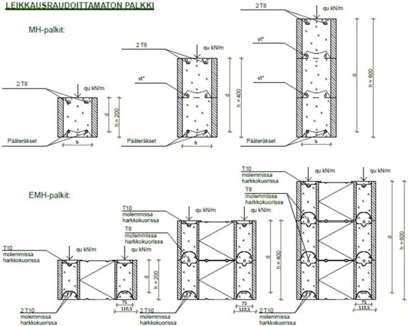
Kuva 2. Leikkausraudoittamaton palkki MH- ja EMH- (EMH-300, EMH-350PRO, EMH-400PRO) harkkoilla. Välisaumojen raudoitus ( vt^* ) asennetaan tarvittaessa ja määritetään tapauskohtaisesti.
