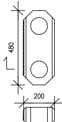
LOHKOMUURIKIVI
