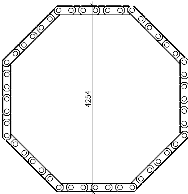
24 reikäkiviparia
