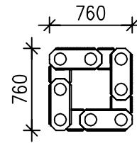
4 reikäkiviparia
