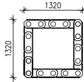
8 reikäkiviparia
