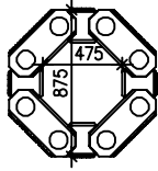
8 reikäkiviparia
