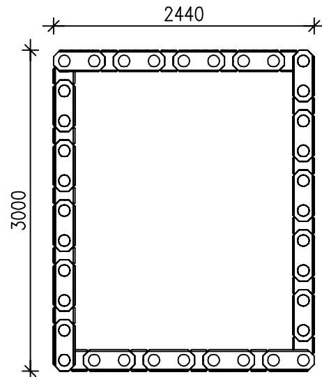
18 reikäkiviparia
