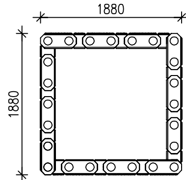
12 reikäkiviparia
