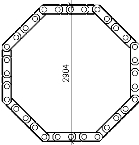
24 reikäkiviparia
