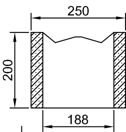
MH-250
