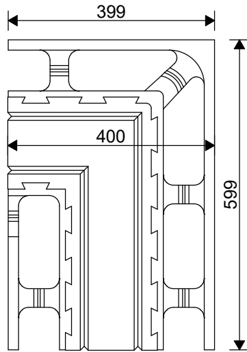
EMH-350PRO KULMA
