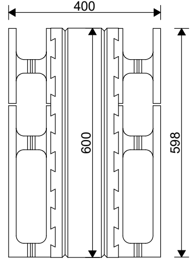
EMH-350PRO PÄÄTY
