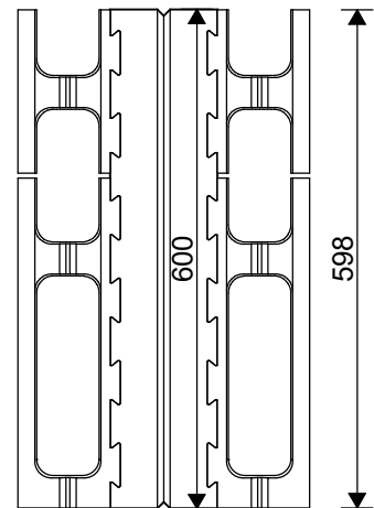
EMH-350PRO PÄÄTY
