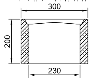
MH-300 PÄÄTYHARKKO
