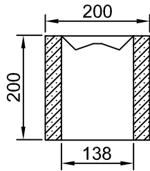
MH-200 PÄÄTYHARKKO
