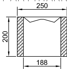
MH-250 PÄÄTYHARKKO
