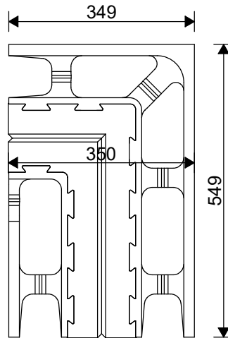
EMH-350PRO KULMA
