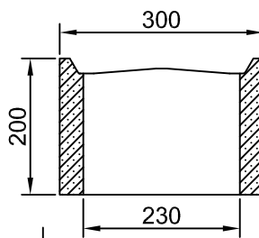
MH-300
