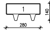
HULEKATUKIVI 80
